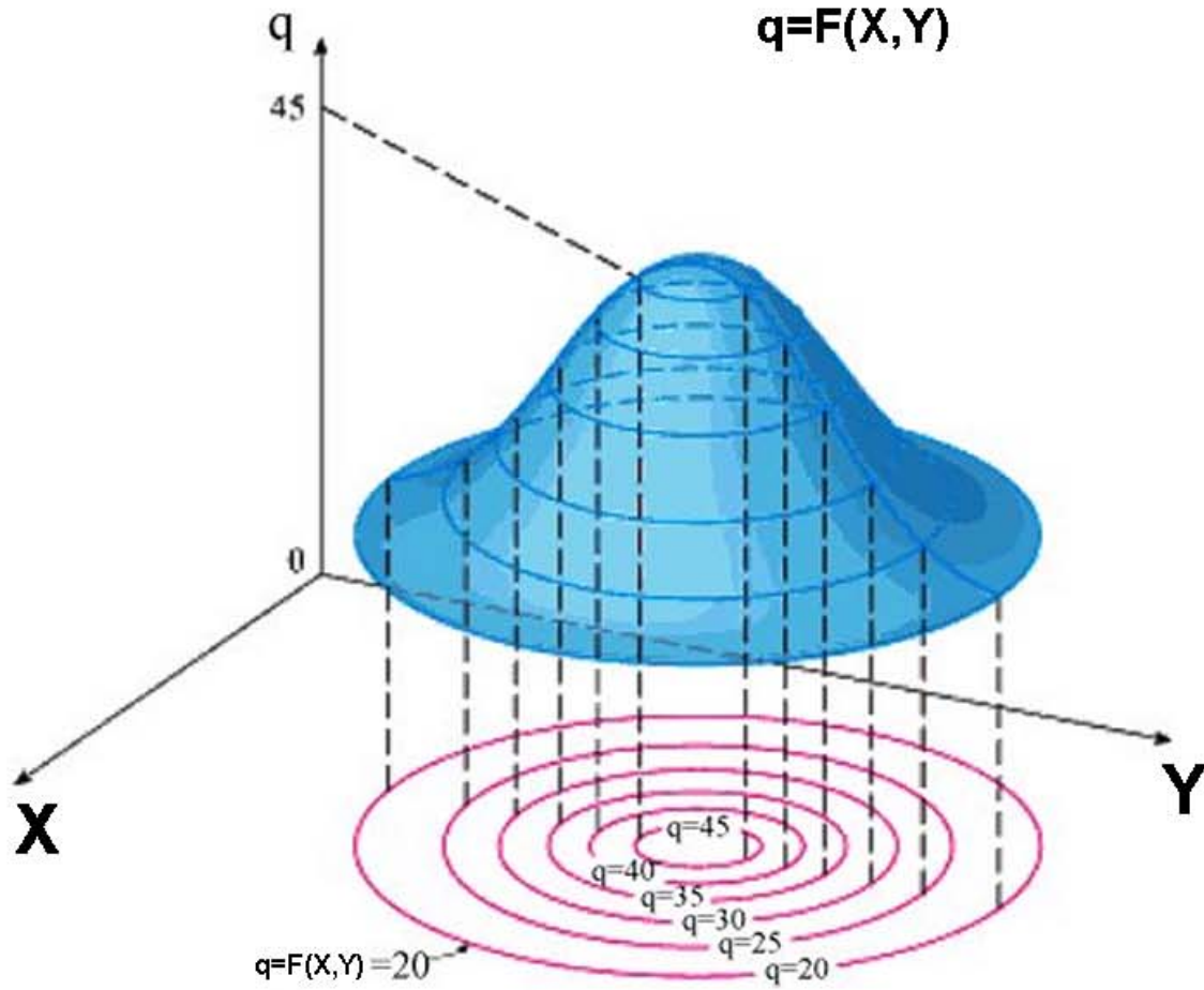
Şekil 1 Eşyükseklik eğrileri
