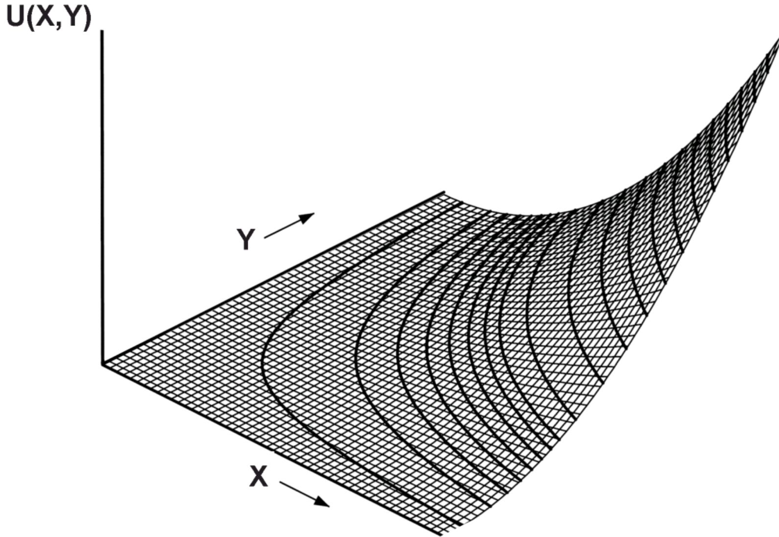
Şekil 2 U(X,Y) = X^2Y^2 Şeklindeki Fayda Fonksiyonu
