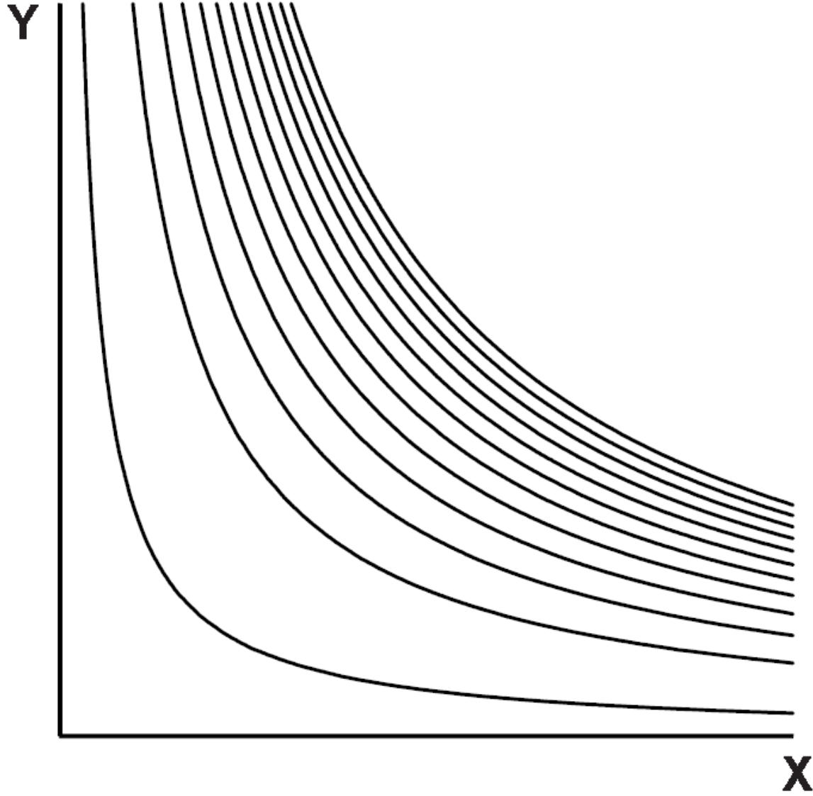
Şekil 9c U(X, Y) = X^2 Y^2 Şeklindeki Fayda Fonksiyonunun Düzey Eğrileri veya Kayıtsızlık Eğrileri
